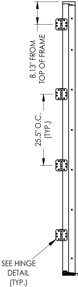
HINGE JAMB
